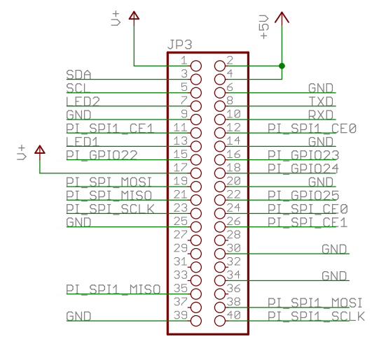
RASPBERRY CON
